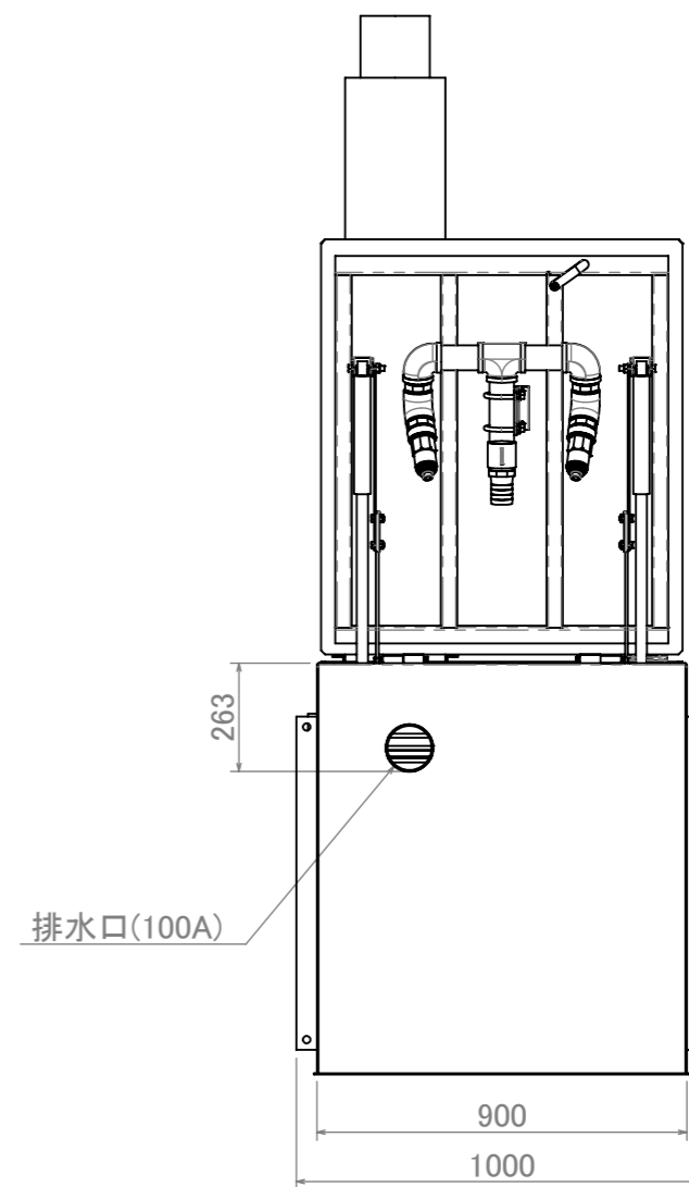
右側面図
