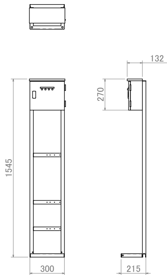
制御盤(操作盤) ※架台付
