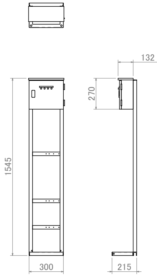
制御盤(操作盤) ※架台付
