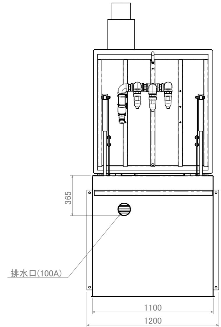
右側面図
