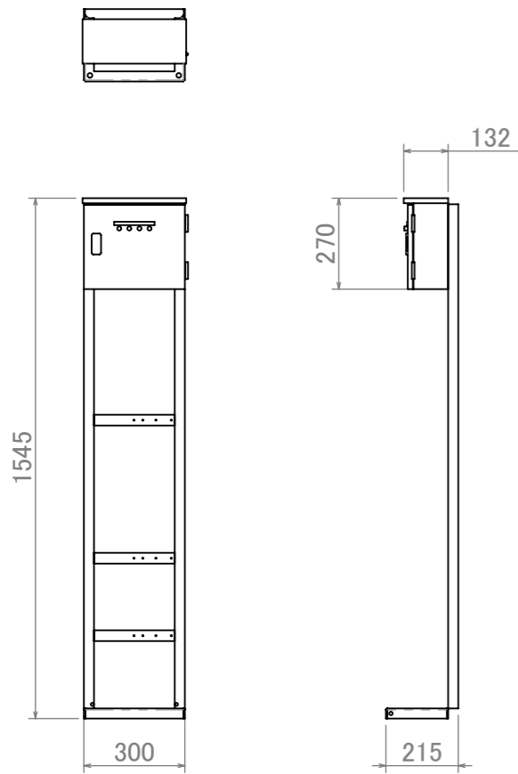
制御盤(操作盤) ※架台付
