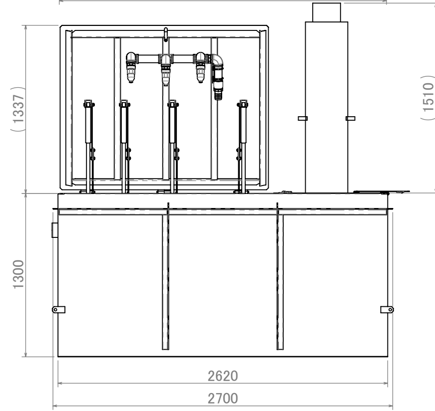
正面図
