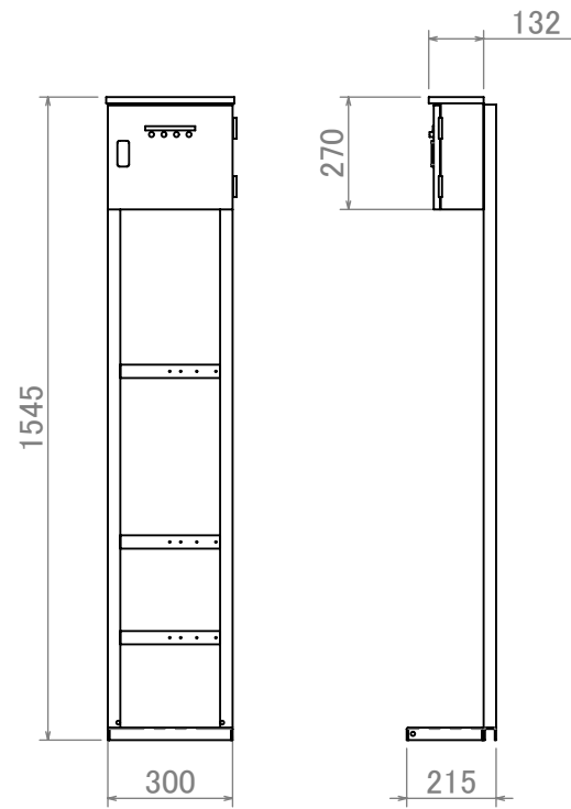
制御盤(操作盤) ※架台付
