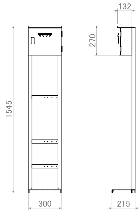
制御盤(操作盤) ※架台付
