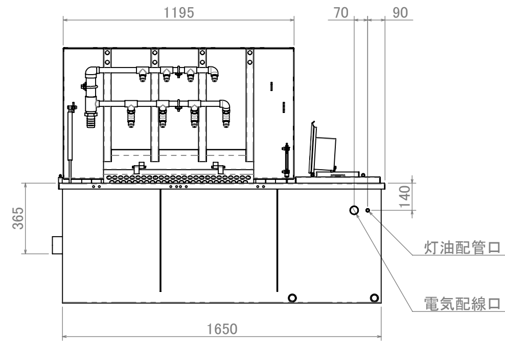
正面図
