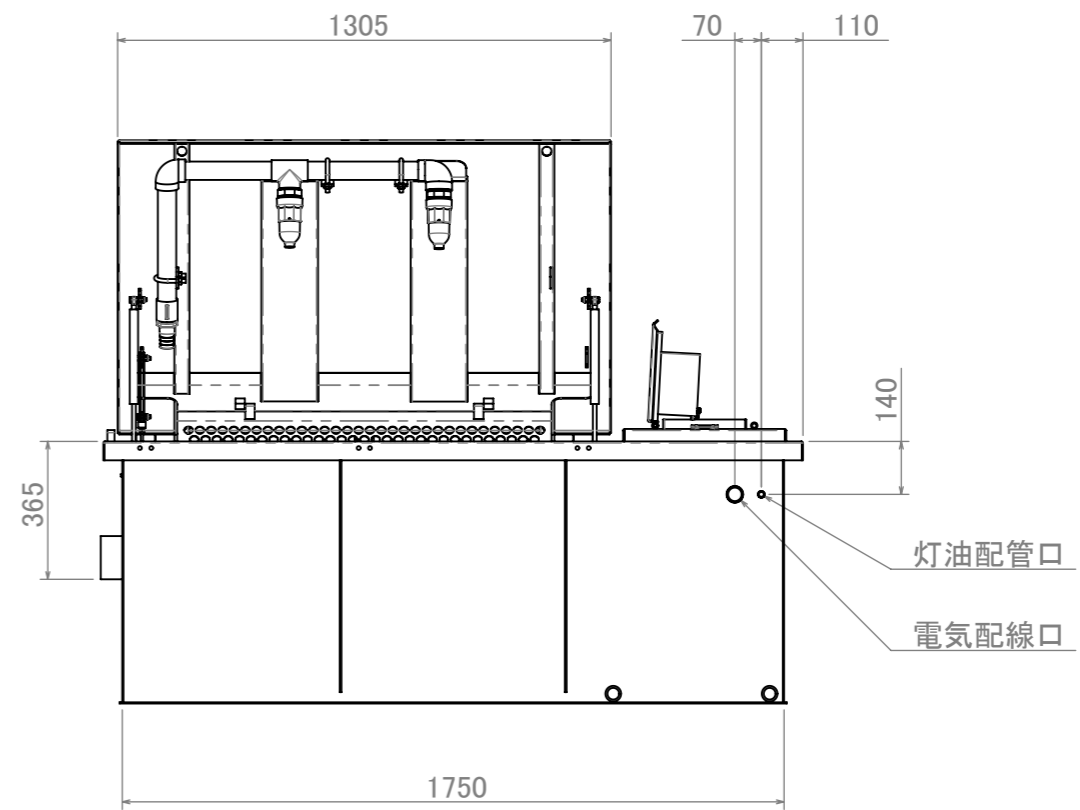
正面図
