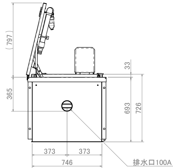
側面図
